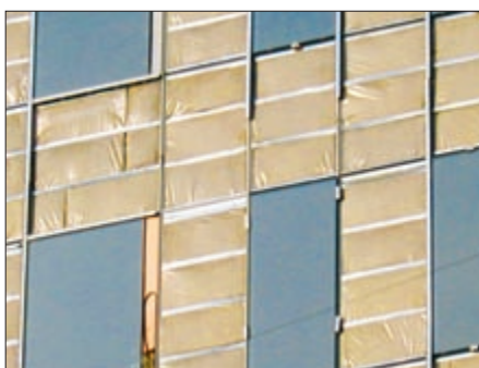
Фото 2. Пример установки полиэтиленовой пленки в качестве ветрозащиты
